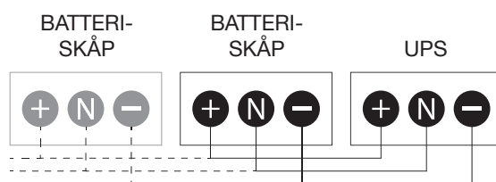
Anslutningsexempel - parallell konfiguration med distribuerat batteri
