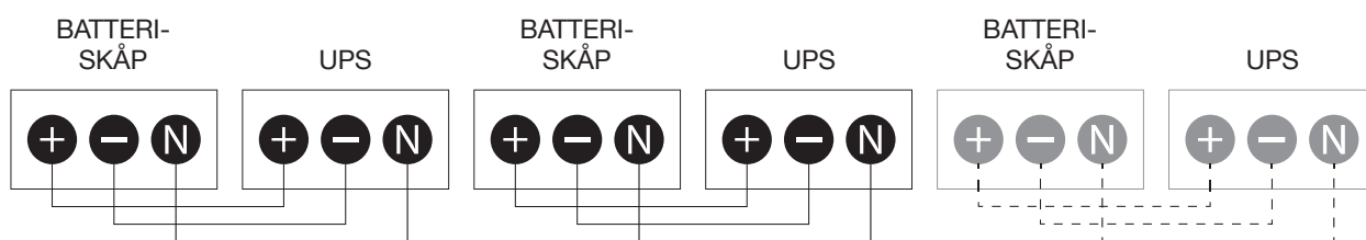
Anslutningsexempel - parallell konfiguration med distribuerat batteri
